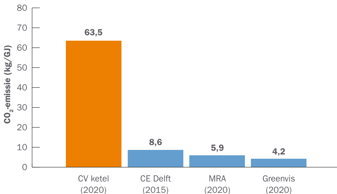
FIGUUR 1 – CO 2 -EMISSION VAN CV-KETEL EN GEOTHERMIEBRON (BEREKEND IN STUDIES CE DELFT, MRA EN GREENVIS)
